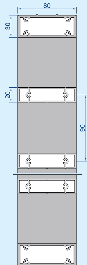
Vertikalschnitt: Maßstab 1:3
