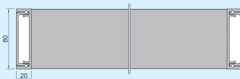
Horizontalschnitt: Maßstab 1:3
