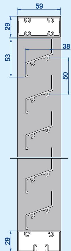
Vertikalschnitt: Maßstab 1:3
