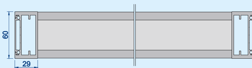
Horizontalschnitt: Maßstab 1:3
