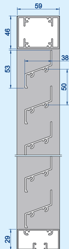
Vertikalschnitt: Maßstab 1:3
