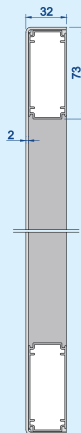
Vertikalschnitt: Maßstab 1:3
