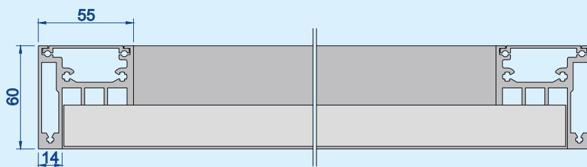
Horizontalschnitt: Maßstab 1:3
