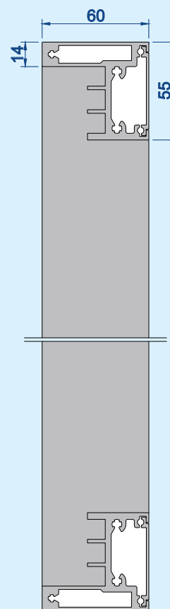
Vertikalschnitt: Maßstab 1:3
