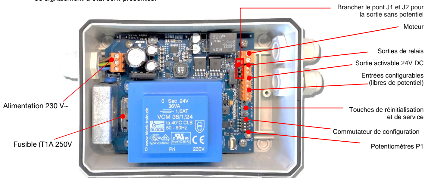
Fig. 1 – Vue de dessus du boîtier électronique
