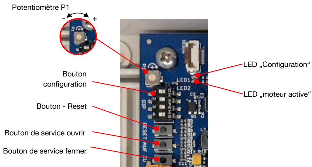
Fig. 2 Potentiomètre, Configuration
