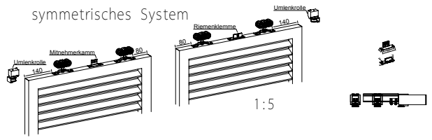
Antrieb
